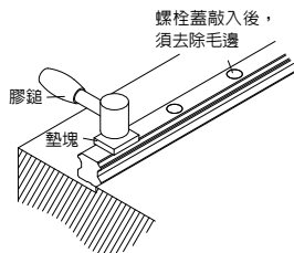
2. 平板墊塊放置於螺栓蓋上，使用膠槌小心將螺栓蓋垂直敲入螺絲孔內，並確保螺栓蓋與滑軌為同一平面高度。(敲入後，螺栓蓋毛邊需去除)
